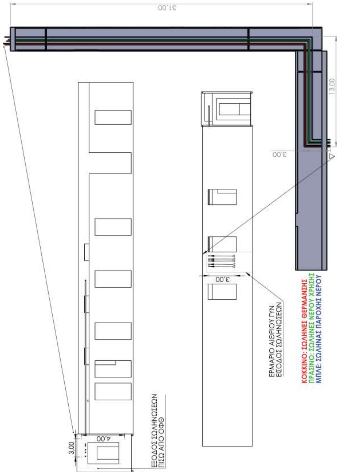
Σχήμα 2: Κάτοψη και όψη των χώρων από τους οποίους διέρχονται οι σωληνώσεις που θα αντικατασταθούν
